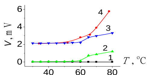
Рисунок 1 - Зависимости ЭДС от температуры структур: pSi-nSi (1), pSi-n(Si 2 ) 1-x-y (ZnSe) x (GaP) y без освещения (2), сумма чистого термо- и фотонапряжения (3) и при освещении солнечным светом (4).
